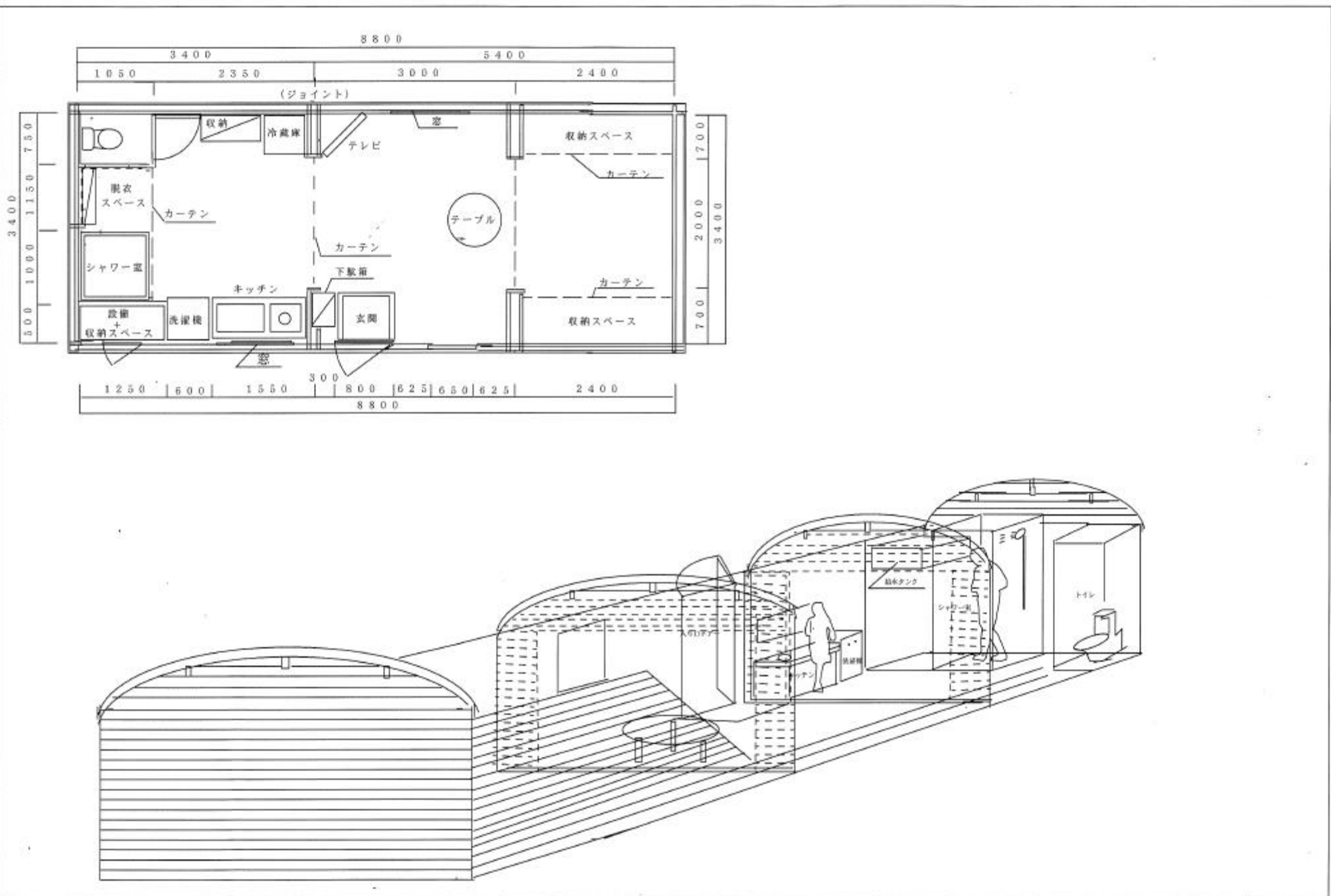
仮設住宅PART 2 (ログ組み立て方式外断熱タイプ)
